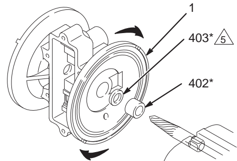
13/32 in EZY-OUT DETAIL VAN VERWIJDEREN LAGER MET EZY-OUT
