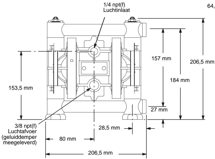
VOORAANZICHT
