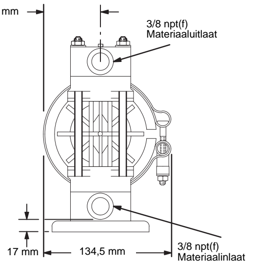
ZIJAAANZICHT
