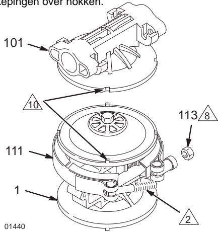
DETAIL VAN KLEMBANDEN EN DEKSELS
