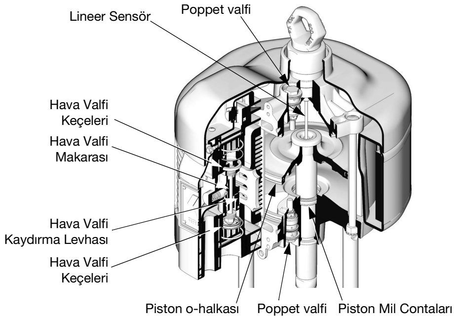
Şekil 7. Kesit Görünüm, Doğrusal Algılayıcı Modeller
