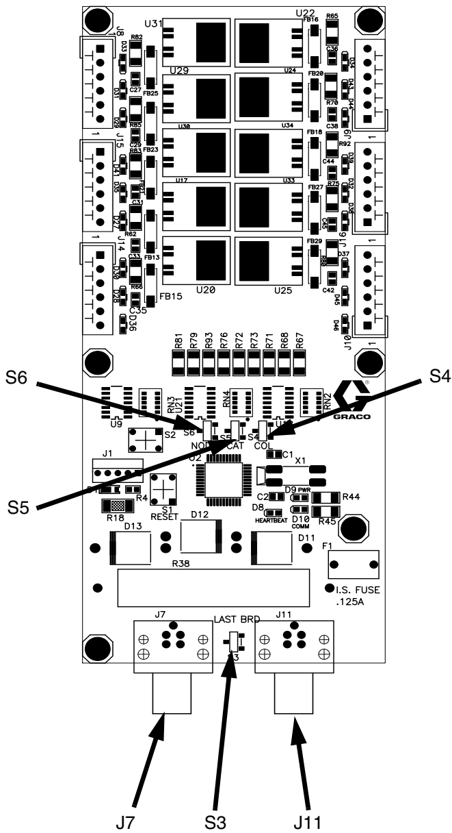
AFB. 16. S3-S6 schakelaars kleurwisselkaart
