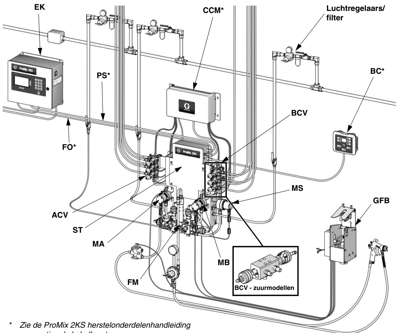
AFB. 2. Manueel systeem, afgebeeld met G3000 meters, kleur/katalysatorwissel, 1 pistoolspoelkast en oplosmiddeldebietmeter (accessoire)
