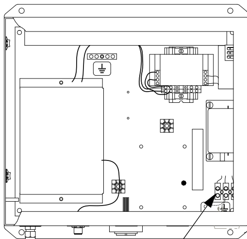
Aansluitblok voor elektrische voeding
