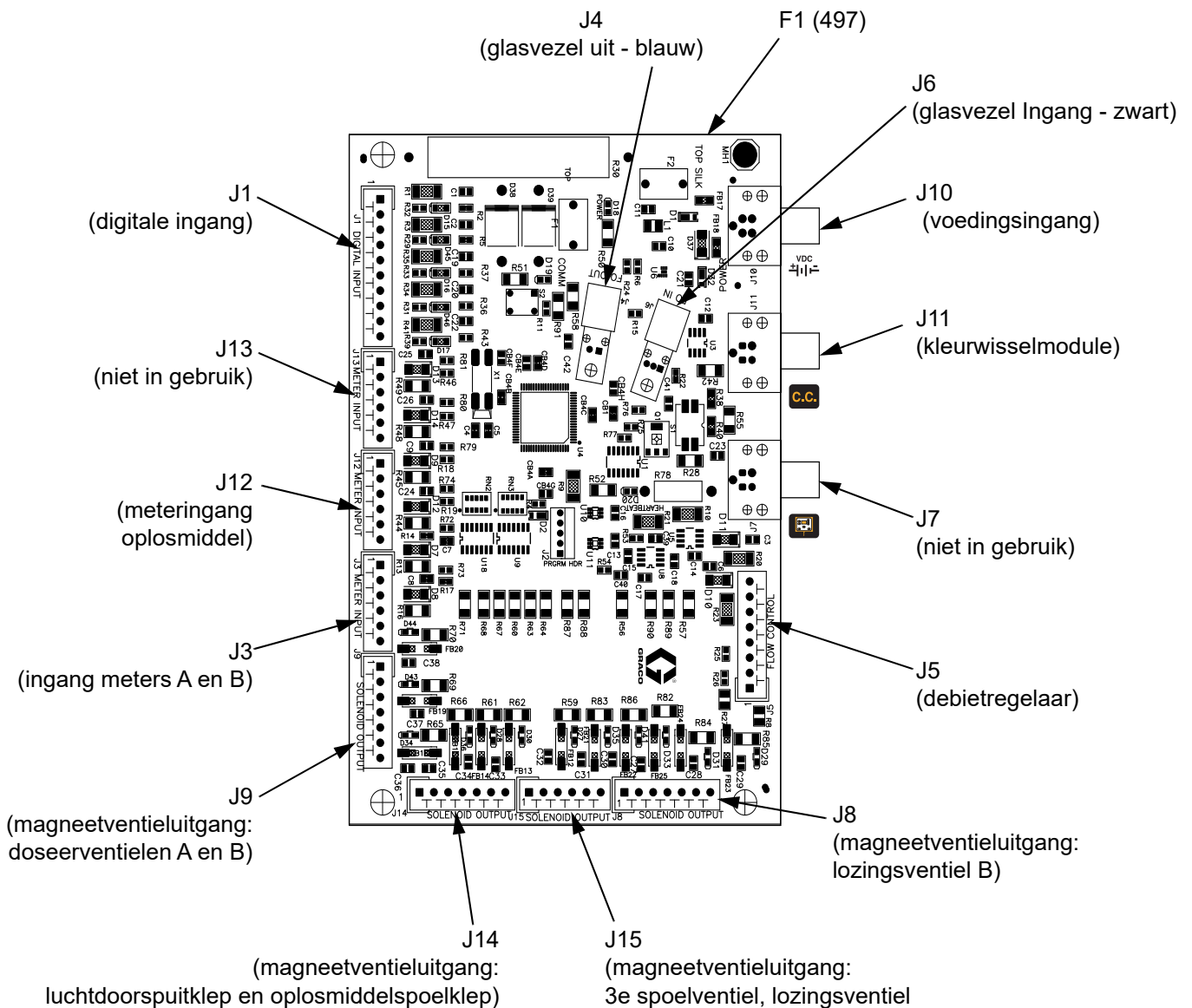
AFB. 29: 255765 Besturingskaart vloeistofstation
