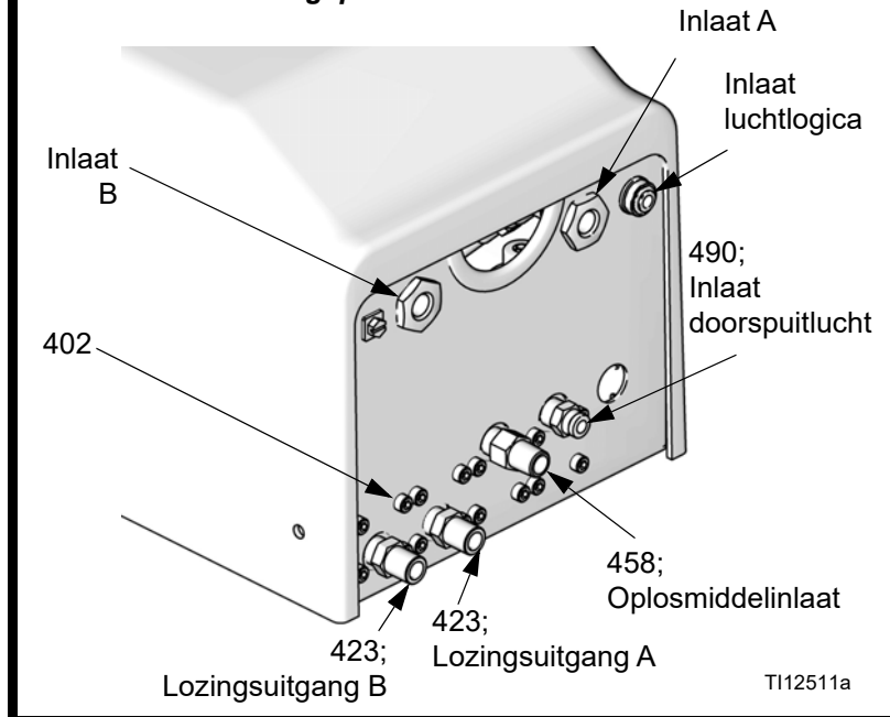
Detail van verbindingsoorten
