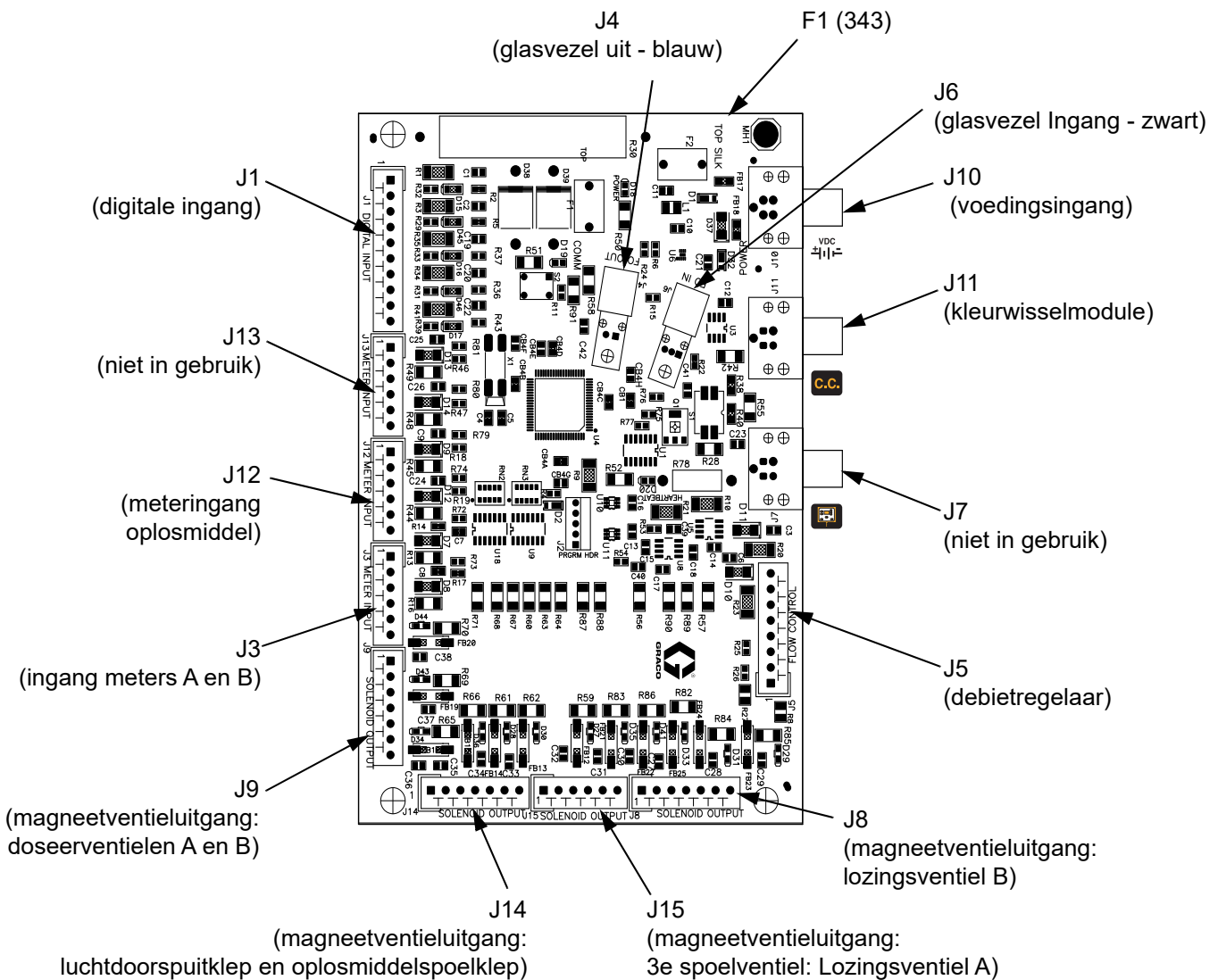
AFB. 21: 255765 Besturingskaart vloeistofstation
