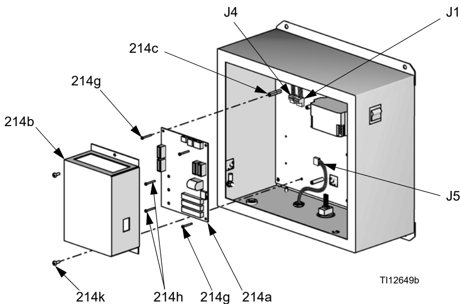
AFB. 17: De barrièrekaart vervangen
