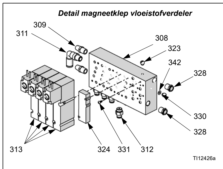
AFB. 20: Wandgemonteerd vloeistofstation
