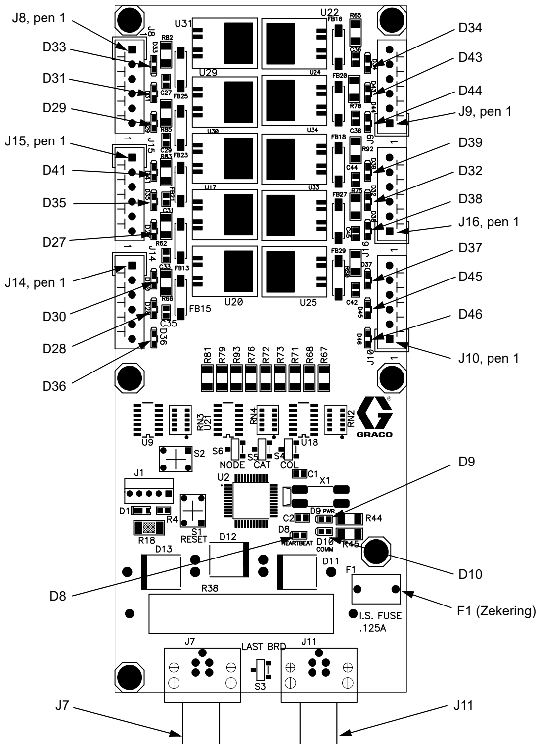
AFB. 13: 256172 kleurwisselkaart
