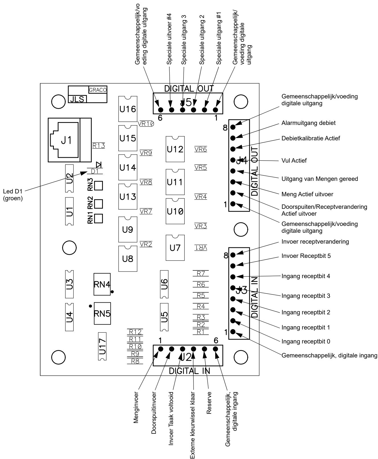
AFB. 10: 255766 Discrete I/O-kaart
