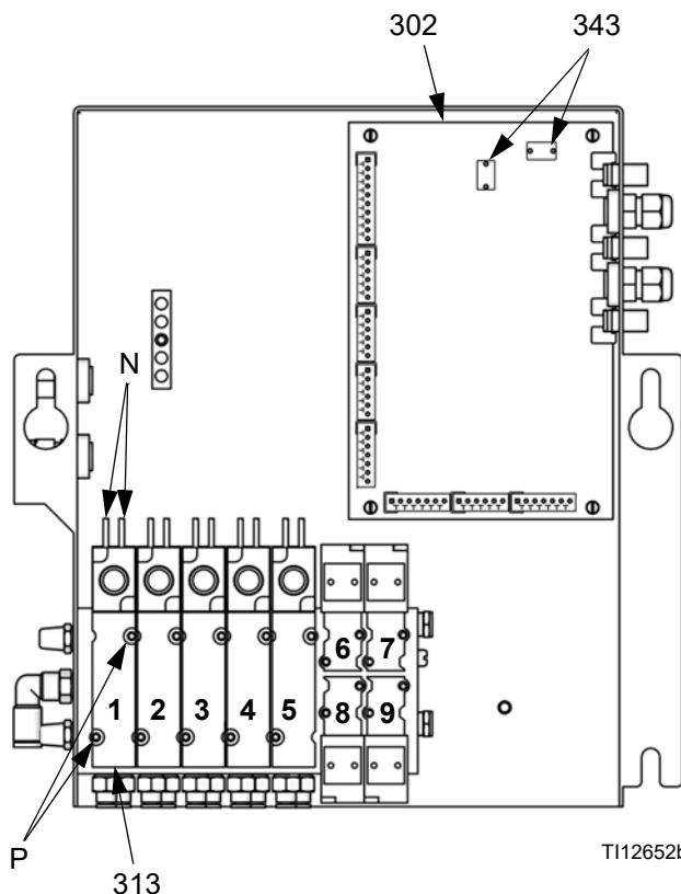
AFB. 22: Magneetventielen en zekeringen vervangen
