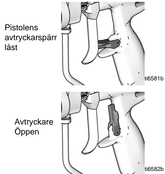
FIG.5. Pistolens avtryckarspärr
