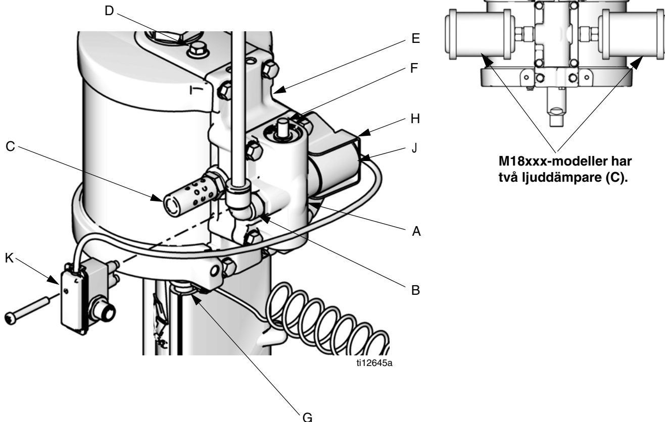
FIGUR 1: NXT luftmotorkomponenter
