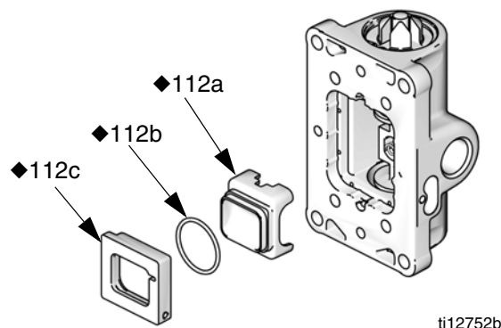
FIGUR 9: Tvådelad koppmontering
