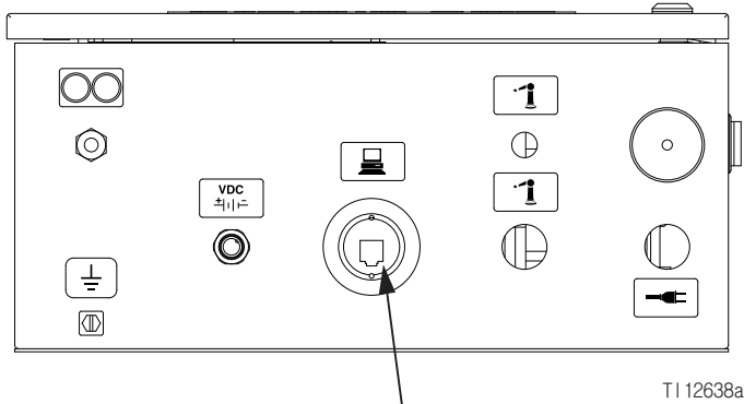
CAT5 케이블 커넥터
