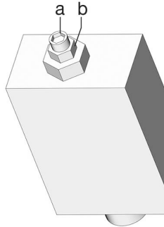
a = Einstellschraube b = Feststellmutter ti15644b
