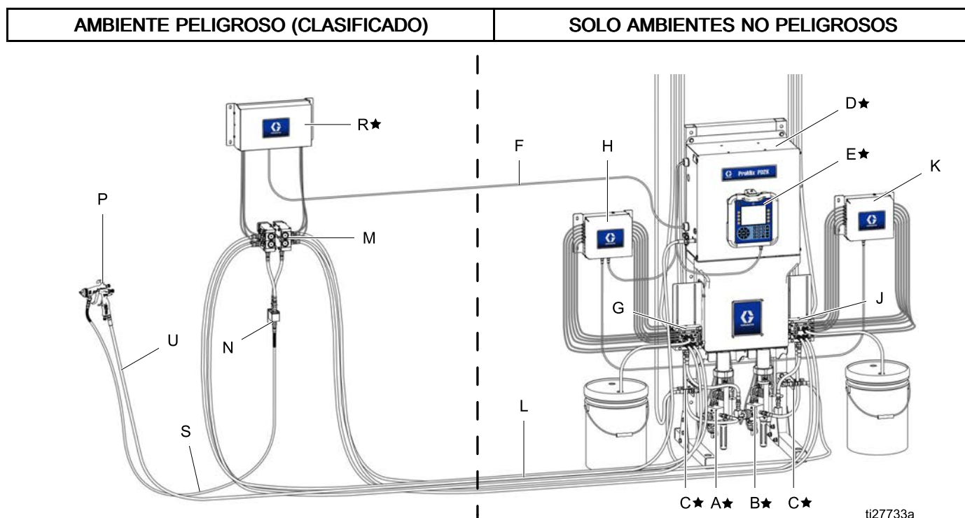
Figure 10 Instalación típica con colector de mezcla remoto
