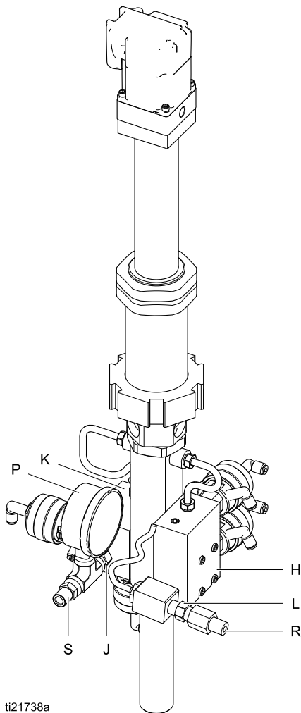
Figure 21 Conexiones de entrada y salida de la bomba
