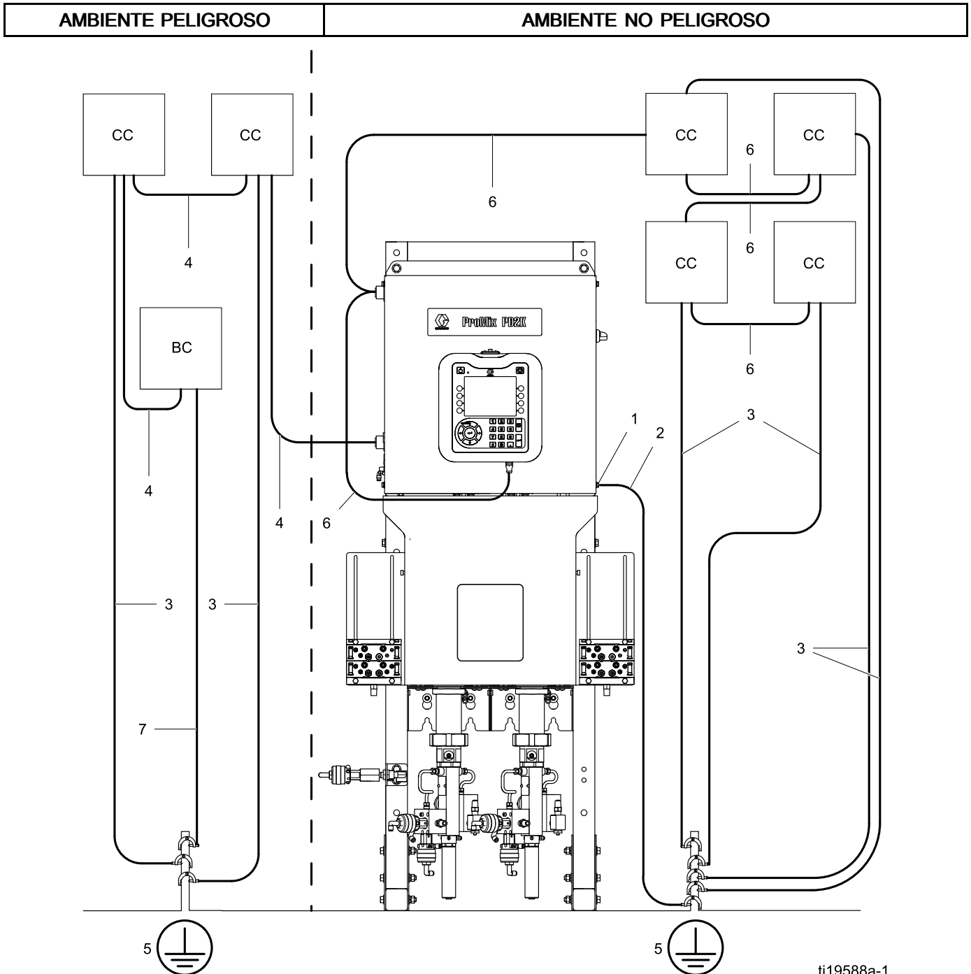
Figure 26 Conexión a tierra del sistema
