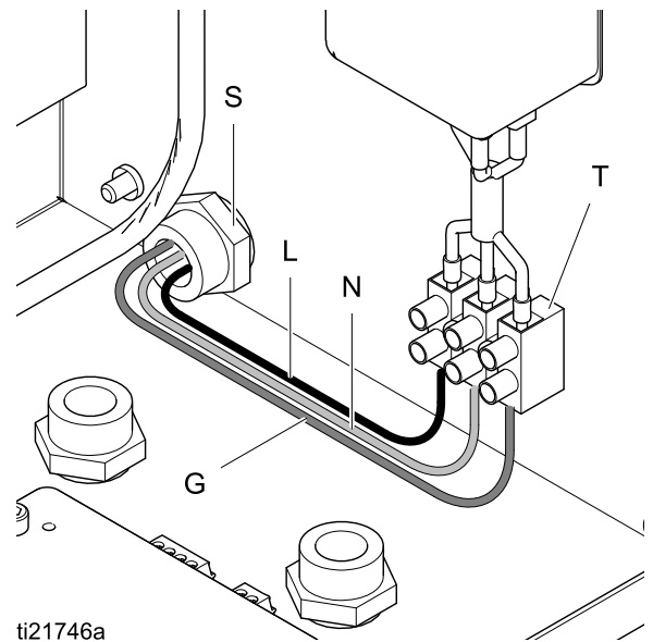
Figure 24 Conexión eléctrica de la caja de control
