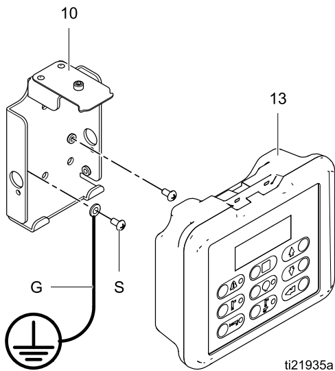
Figure 17 Conecte a tierra la ménsula del control de cabina
