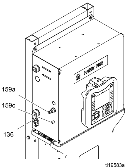
Figure 19 Conecte el aire de atomización
