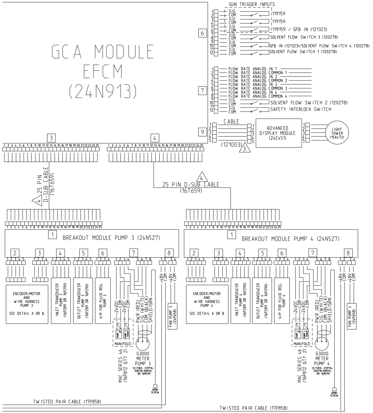
Figure 29 Esquema eléctrico, hoja 2, parte 2 CONTINÚA EN LA PÁGINA SIGUIENTE
