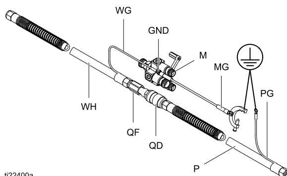
Figure 23 Kit de desconexión rápida de manguera de aire electrostática
