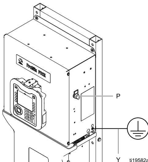
Figure 25 Tornillo de conexión a tierra e interruptor de alimentación
