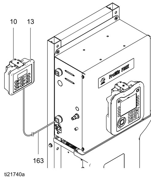
Figure 18 Instalación del control de cabina
