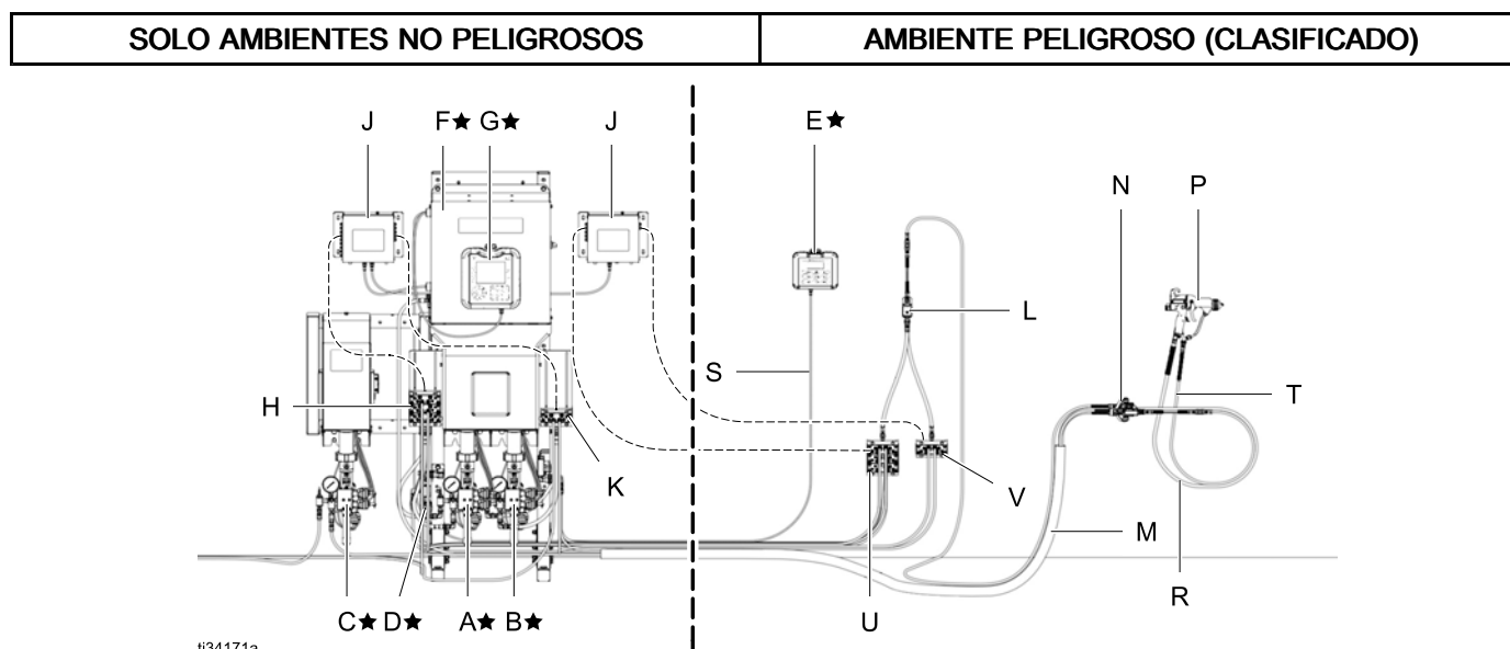
Figure 12 Instalación típica de PD3K+ (MC1000, MC2000, MC3000, MC4000)
