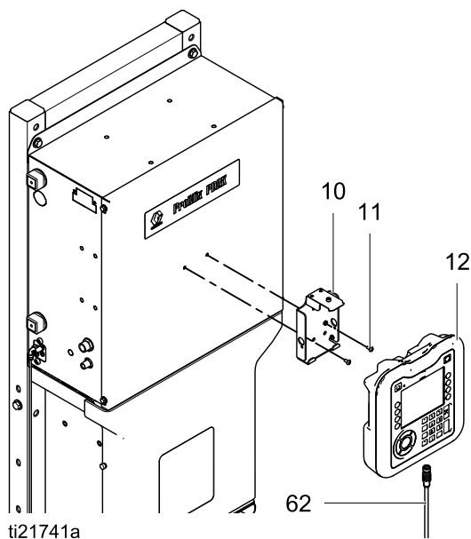
Figure 13 Instalación del módulo de pantalla
