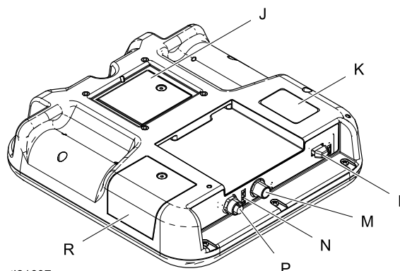
Figure 14 Puertos de conexión del módulo de pantalla avanzada
