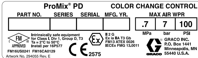
Figure 5 Etiqueta de identificación de Control de cambio de color intrínsecamente seguro (accesorio)
