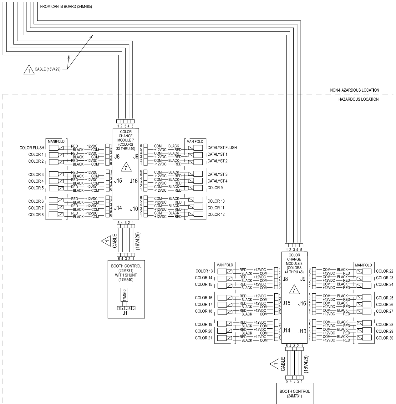
Figure 37 Esquema eléctrico, hoja 3, parte 2 CONTINÚA EN LA PÁGINA SIGUIENTE
