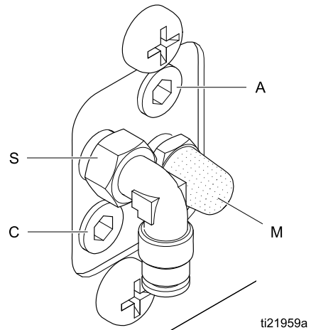
Figure 20 Conexiones del colector de aire
