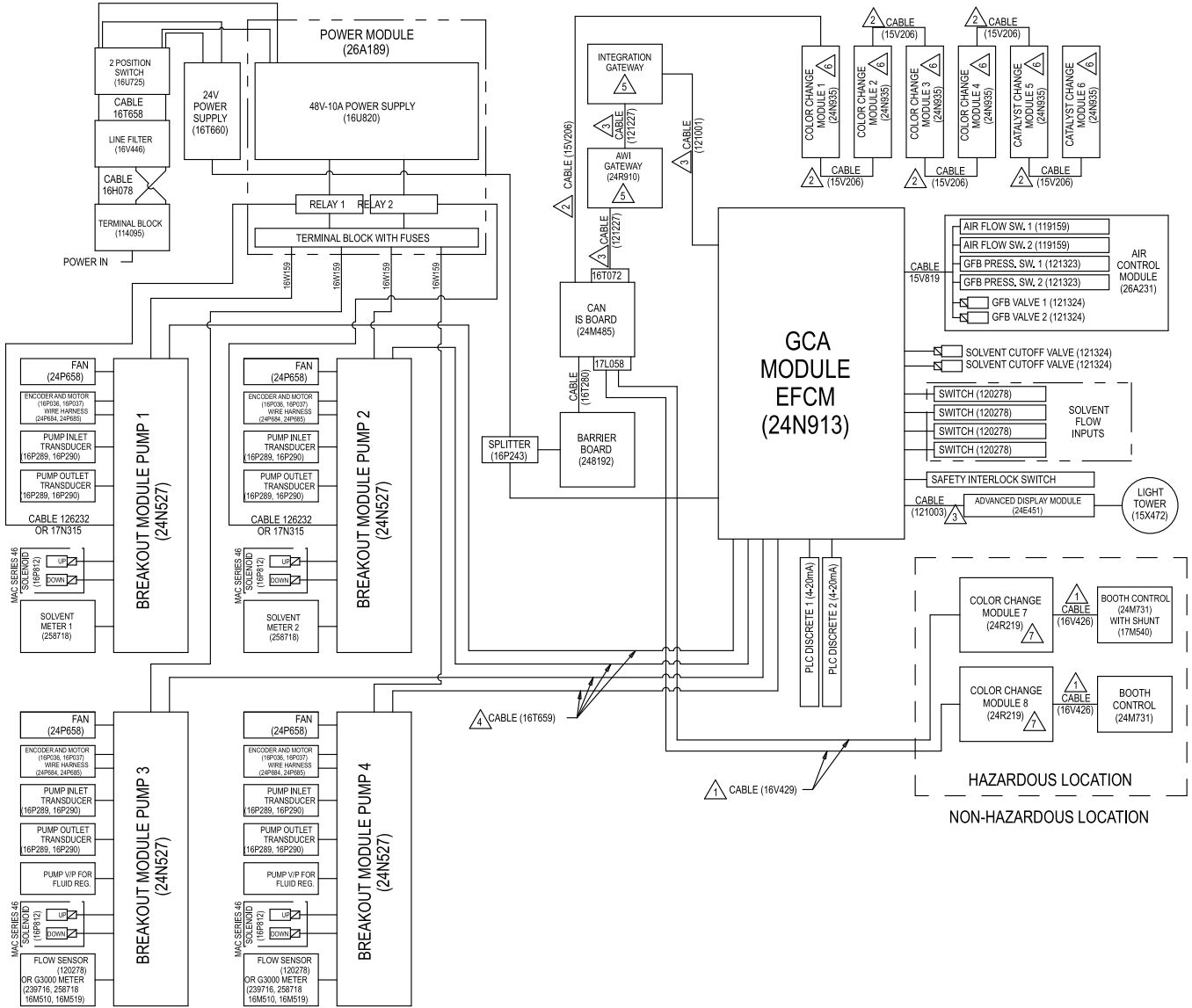
Figure 33 Esquema eléctrico, hoja 1
