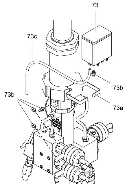
Figure 22 Instalación del kit de recipiente TSL
