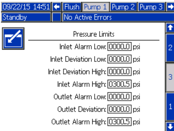
Figure 61 Pantalla de bomba 3, Supervisión de presión habilitada
