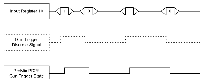
Figure 14 Sincronización de gatillo de pistola (se muestran las señales discretas y de red)
