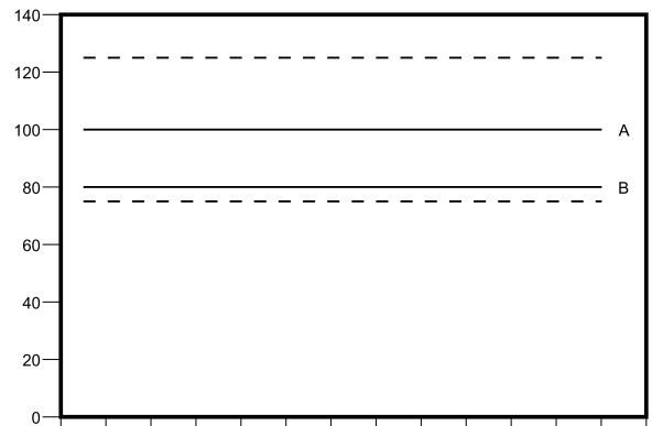
Figure 43 El rango de presión de salida aceptable de la bomba B para un sistema con un objetivo de presión de pulverización (A) de 100 psi y una tolerancia de presión de mezcla del 25 %.
