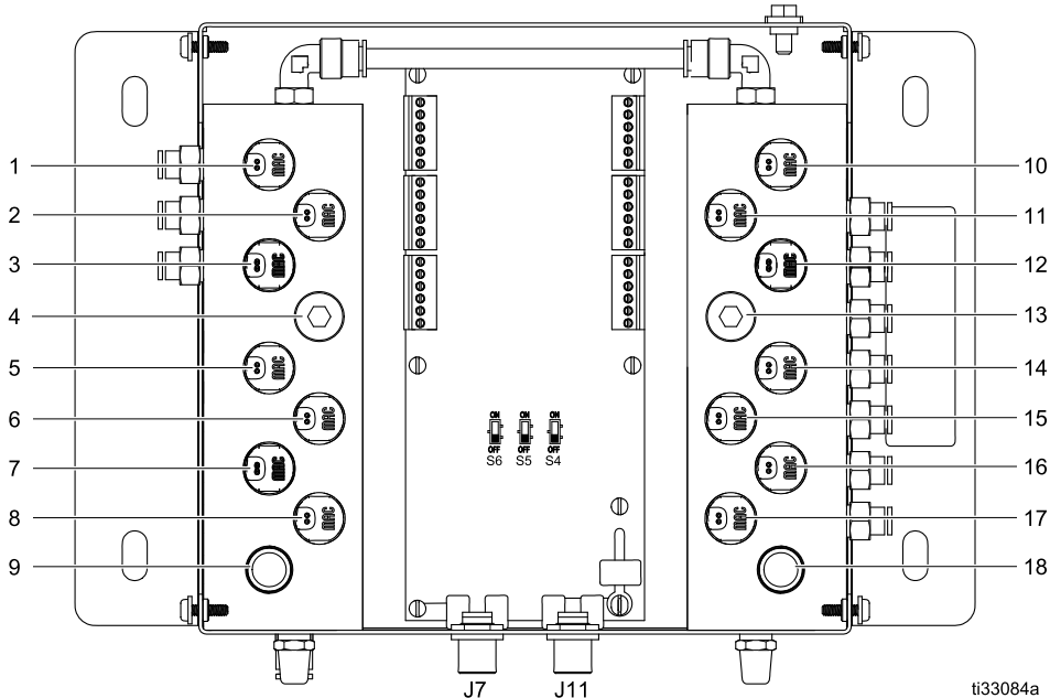
Figure 53 Enumeración de ubicación de solenoides
