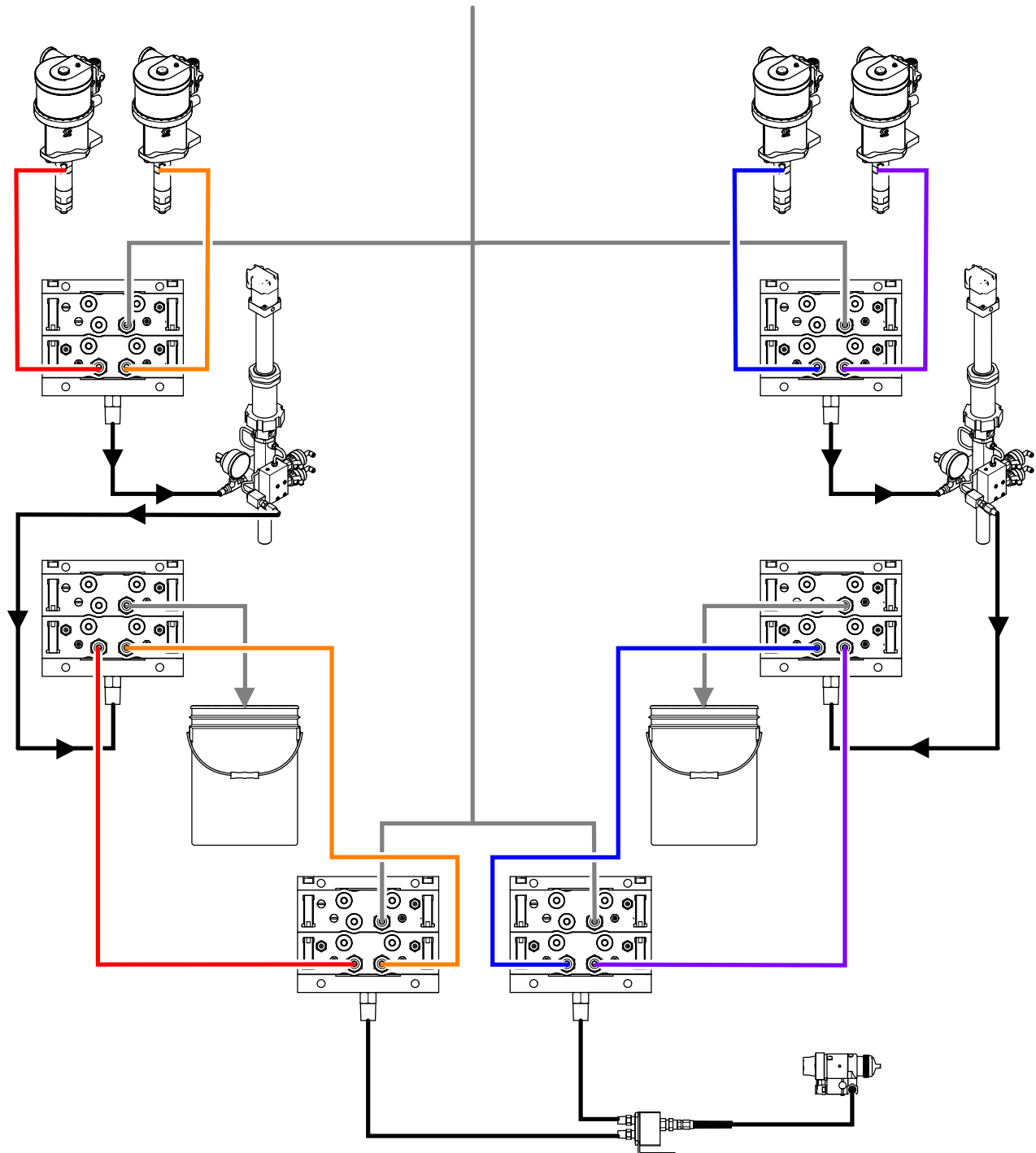
Figure 85 Líneas de fluido para un sistema automático PD2K normal.
