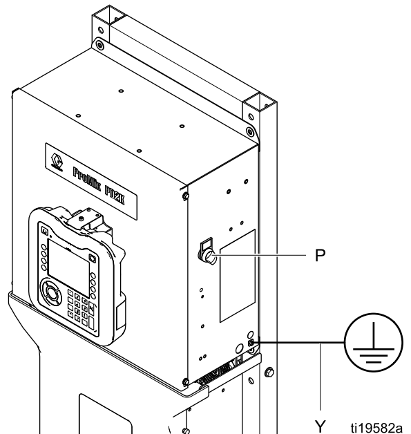
Figure 10 Interruptor de alimentación
