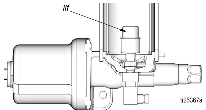
Fig. 9: Galleggiante basso livello in posizione sollevata
