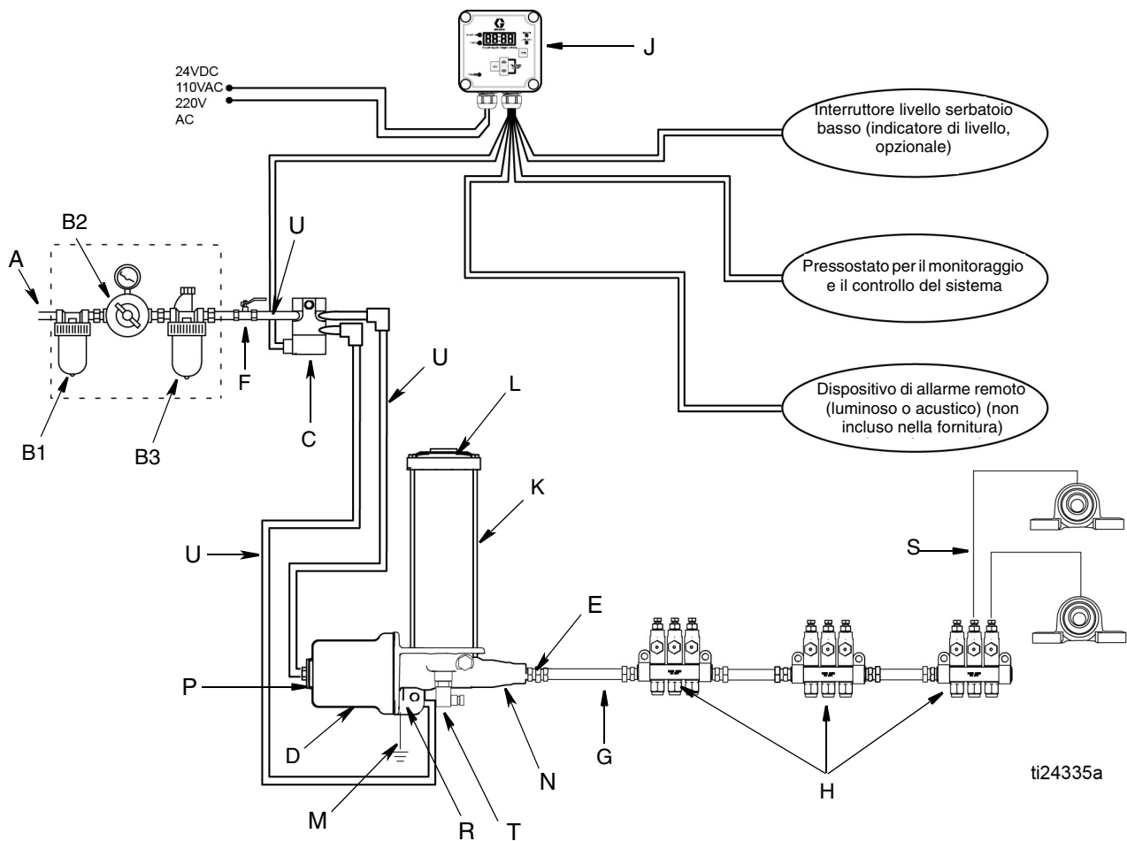
FIG. 1: Installazione tipica
