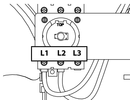
Рис. 11. Показана система 230 В, 1-фазная
