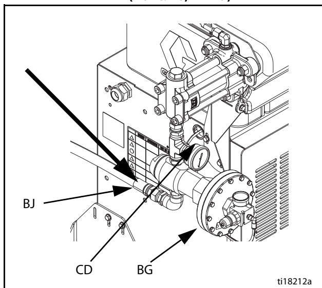
Вход материала системы HFRS (макс. 20,7 МПа)
