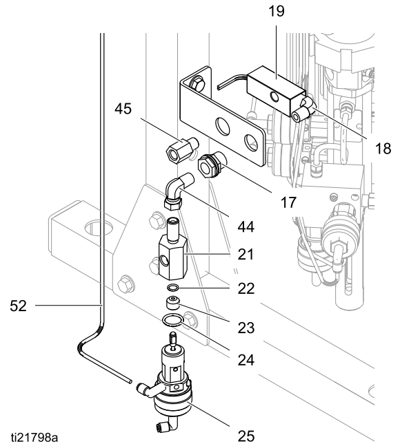
Figure 49 Oplosmiddelventiel en oplosmiddelstromingsschakelaar
