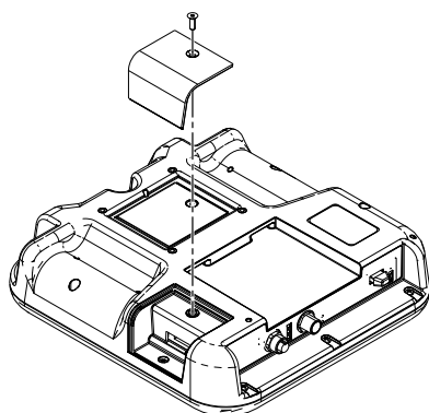
Figure 33 Tokentoeegangspaneel verwijderen
