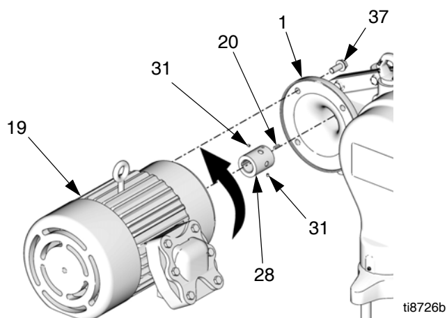
FIG. 22. Tous les moteurs électriques sur châssis 182/184 TC NEMA
