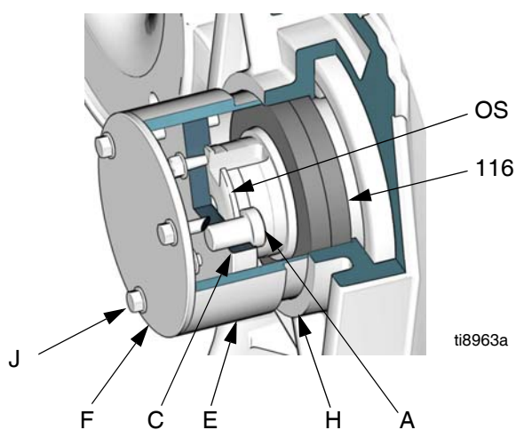
FIG. 28 : Kit de joints du démultiplicateur
