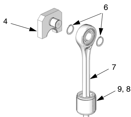
FIG. 21. Bras de manivelle et tige de connexion
