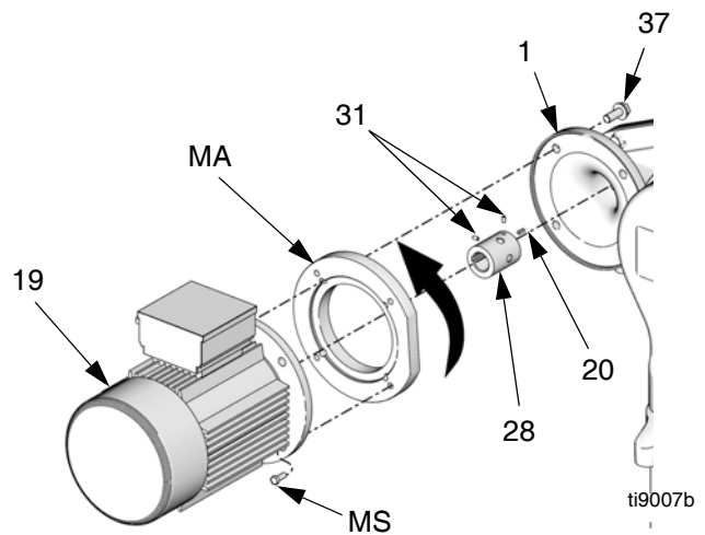
FIG. 23. Moteurs électriques sur châssis IEC 112M/B5 et 100L/B5
