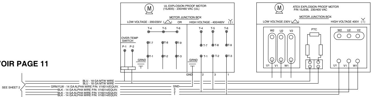
Schéma des commandes de l'IS 288110
