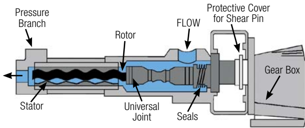
Rotor
