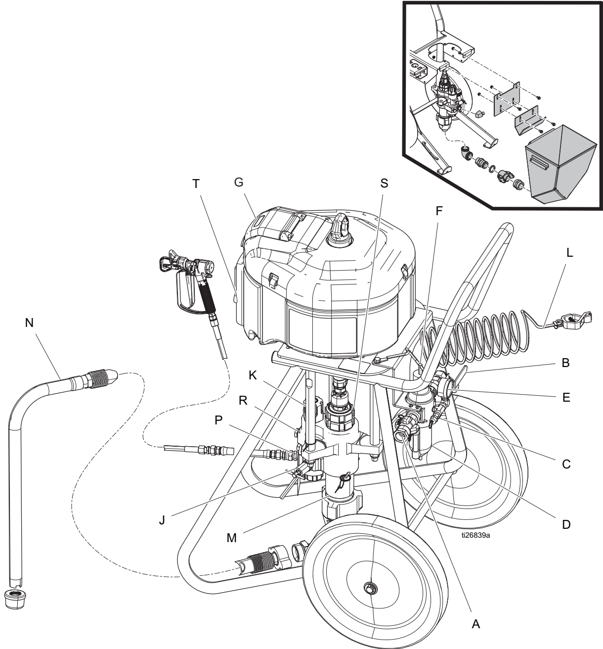
그림 1: 에어리스 도장기
