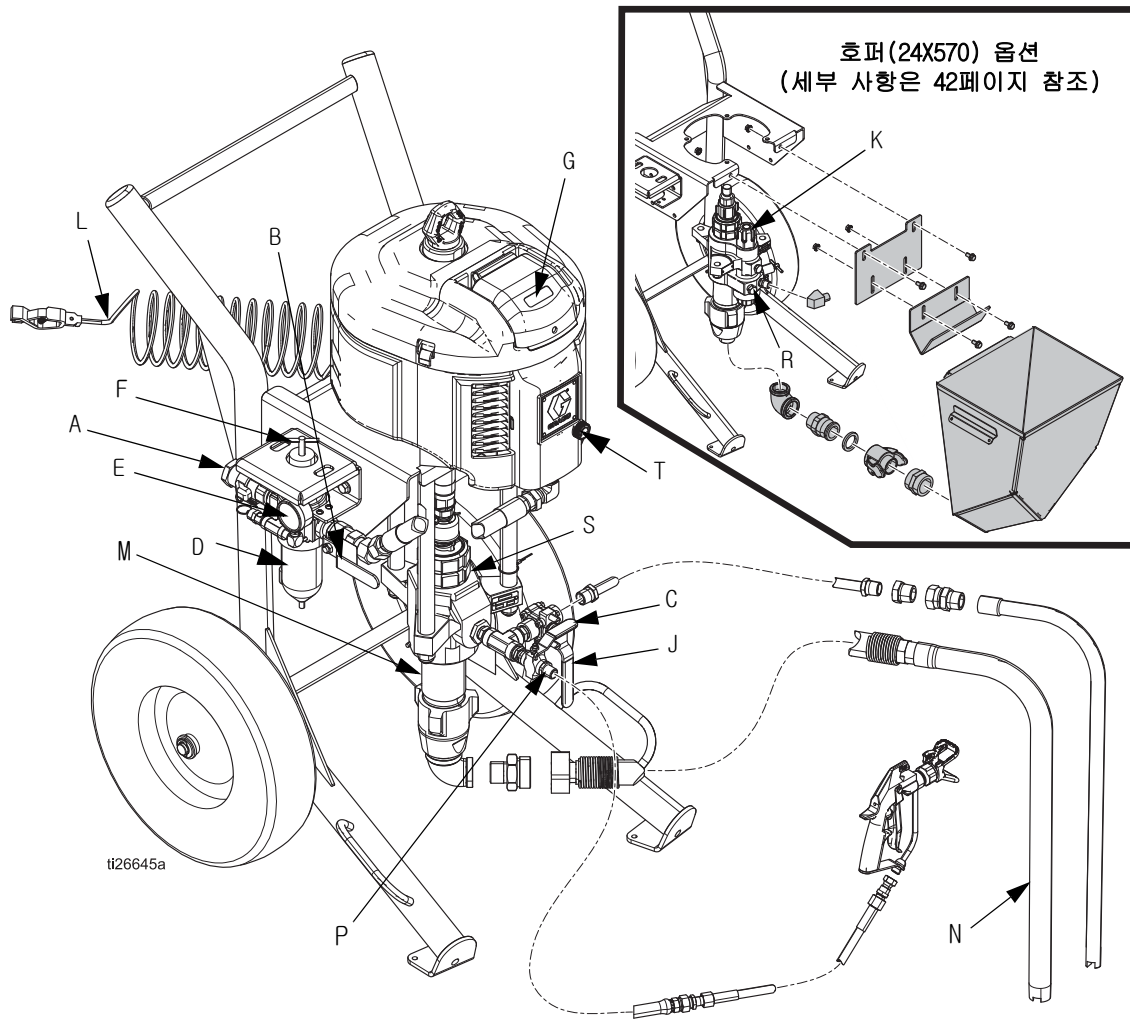
그림 2: 에어리스 도장기
