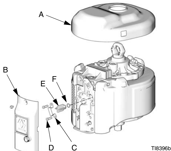
FIG. 2. Desmontaje
