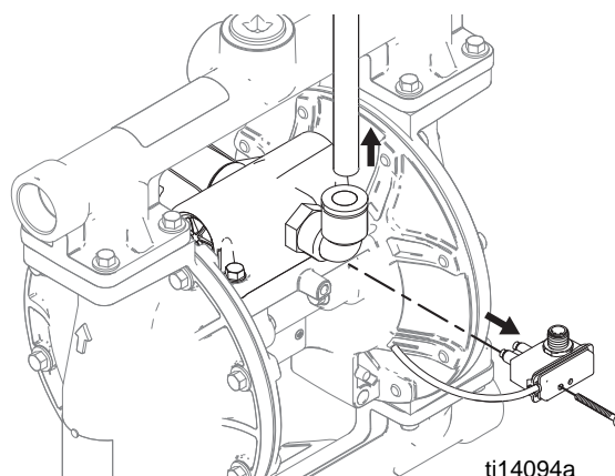
ti14094a Fig. 1. Conjunto del interruptor de lengüeta y extracción de la línea de aire
