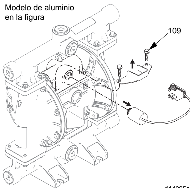
ti14095a Fig. 2. Extracción del solenoide
