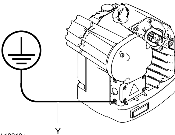
Figure 8 接地線
