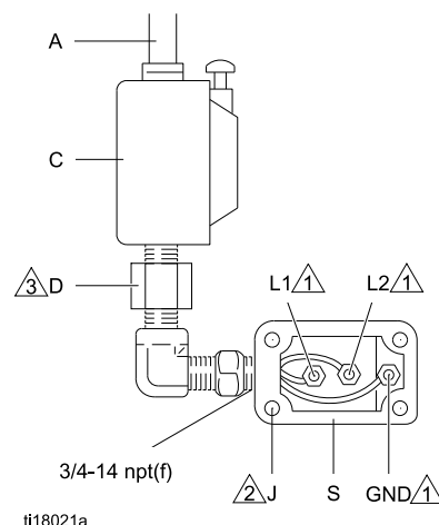
Figure 7 Anslut strömkablar
