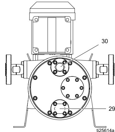
Figure 1 Aftapgat (29) en ontluchtingsgat (30) van de pomp
