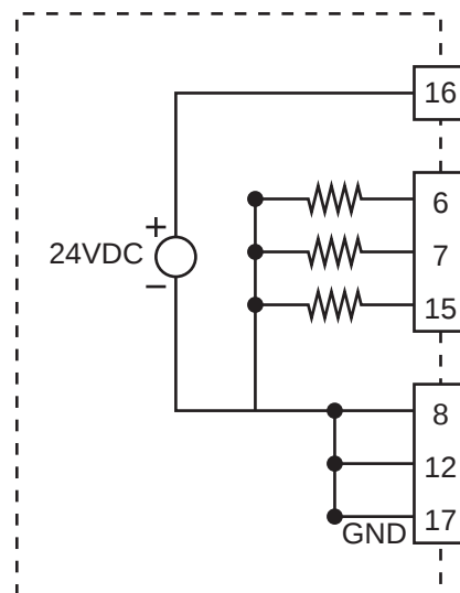
Figure 4 Wyjścia cyfrowe – tryb zasilania
