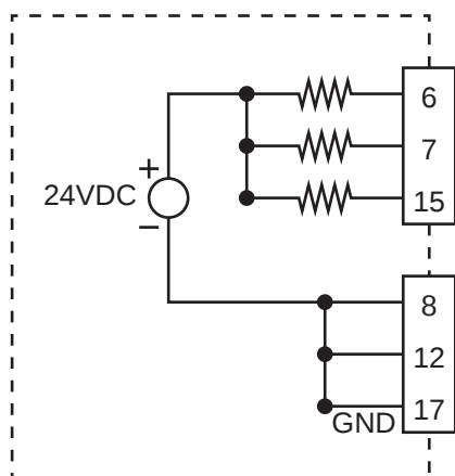
Figure 3 Wyjścia cyfrowe – tryb obciążenia
