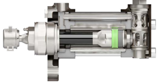
Elite Teknolojisine Sahip Z-Pompasının Bir Kesiti
