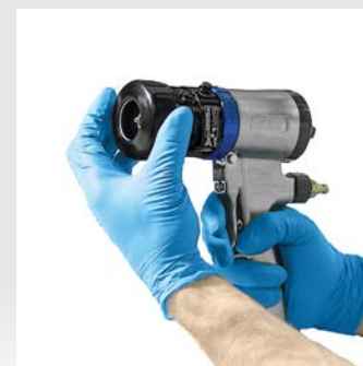
Plaats de borgring en de luchtkap
