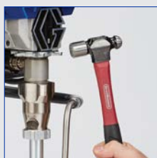
Løsn spændemøtrikken
