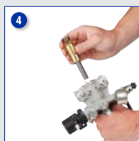
4 Installare la nuova cartuccia e riposizionare la pompa
