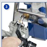
3 Usare la sezione esagonale del telaio per allentare la pompa e rimuovere la cartuccia
