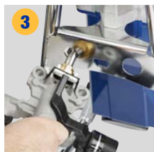
3 Используйте шестигранный разъем на раме для извлечения картриджа
