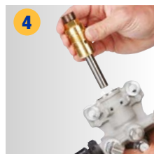
4 Установите новый картридж и замените насос
