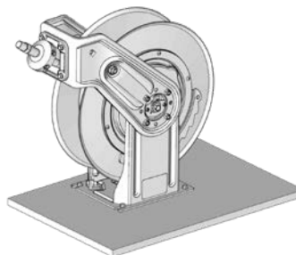
Montage sur table de travail / camion
