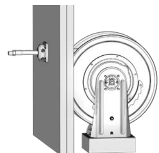
Montage sur camion avec guide de rouleau monté à distance
