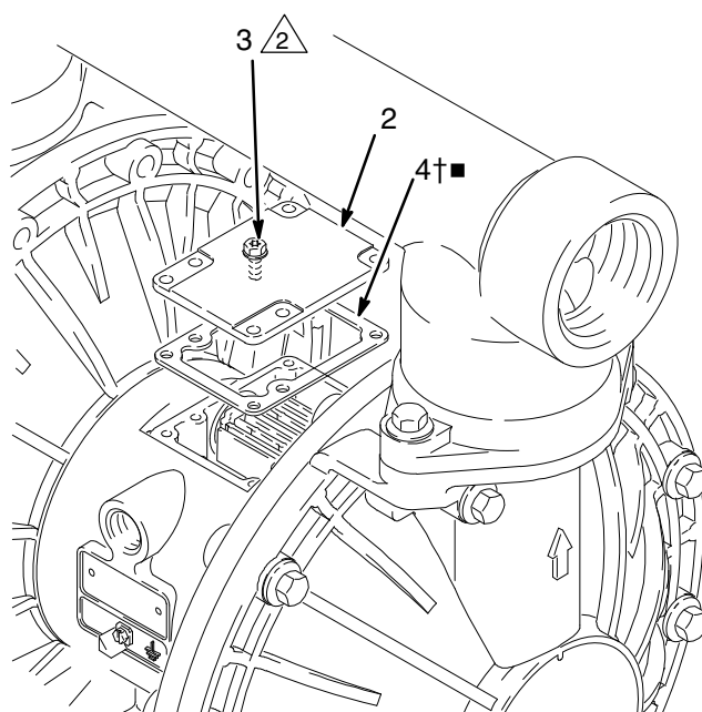
2 Dra åt till moment 5,6 till 6,8 Nm (50-60 tum-lb).
