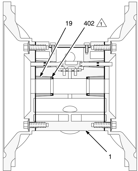
Genomskärning med membranen borttagna
