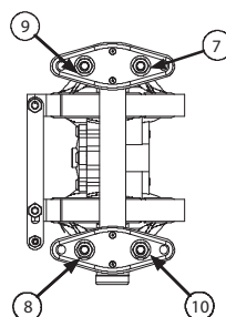
VY UNDERIFRÅN
