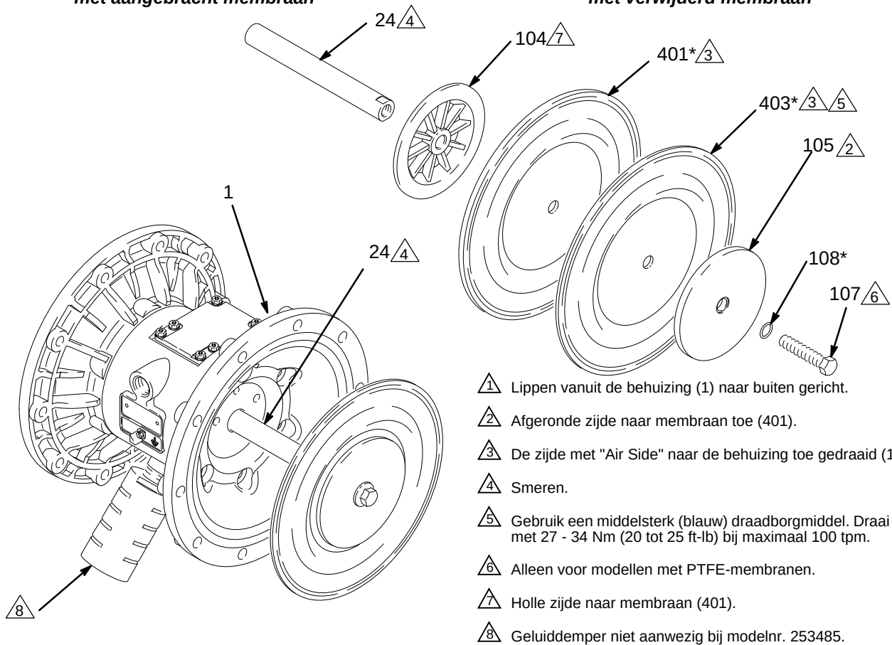
Opengewerkte tekening, met aangebracht membraan
