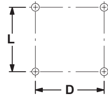
DISPOSIZIONE DEI FORI DI MONTAGGIO DELLA POMPA
