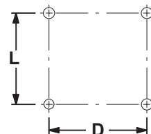
MÖNSTER FÖR MONTERINGSHÅL FÖR PUMP
