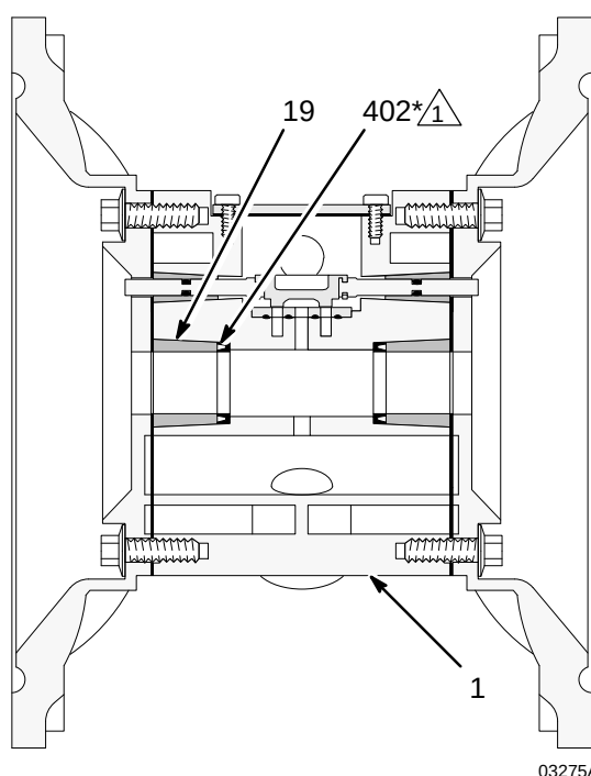
Genomskärning med membranen borttagna
