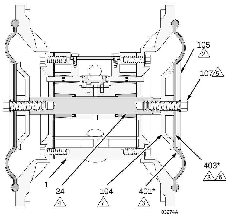
Genomskärning med membranen på plats
