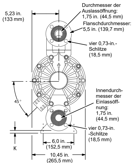
SEITENANSICHT
