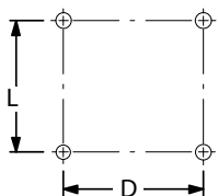
VORLAGE DER MONTAGEBOHRUNGEN
