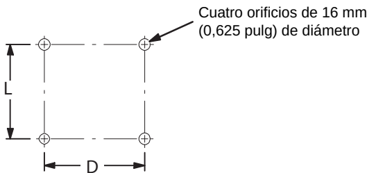
DISPOSICIÓN DE LOS ORIFICIOS DE MONTAJE DE LA BOMBA
