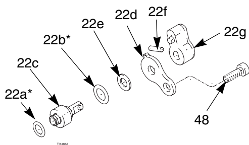
Pos. 22: Válvula ES ON/OFF
