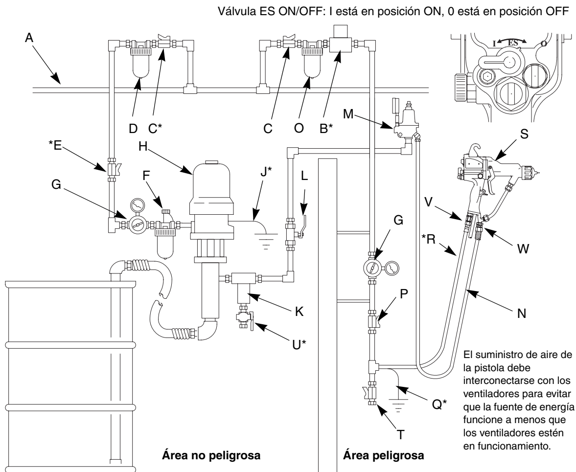
Fig. 2. Instalación típica
