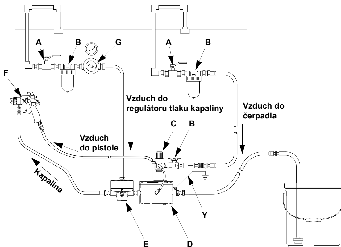
Obr. 5. Nízkotlaký necirkulující systém s pneumatickým regulátorem tlaku kapaliny
