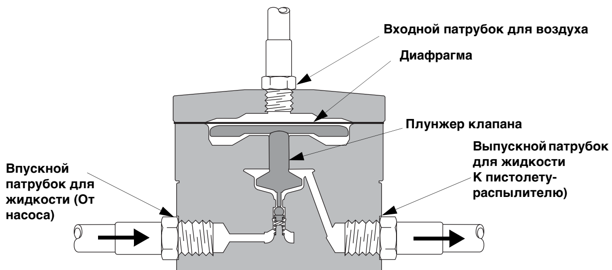
Рис. 2. Вид в разрезе механического регулятора давления жидкости
