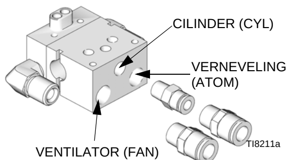
FIG. 2: Luchtfittingen
