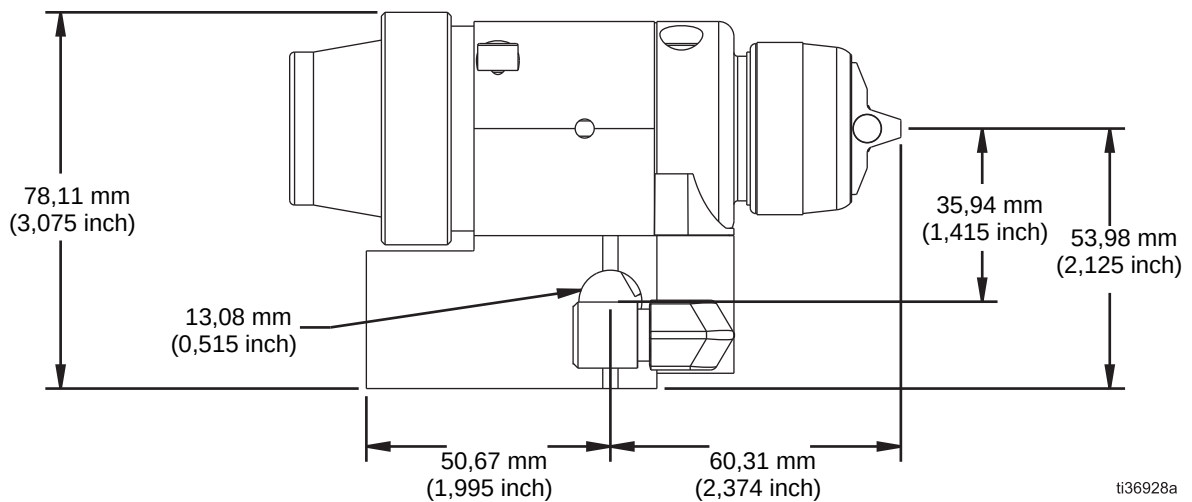
FIG. 30: Ontwerp van de bevestigingsgaten
