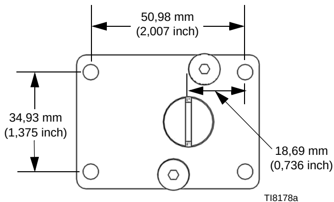
FIG. 26: Ontwerp van de bevestigingsgaten
