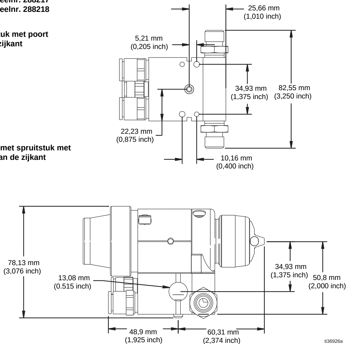
FIG. 28: Ontwerp van de bevestigingsgaten
