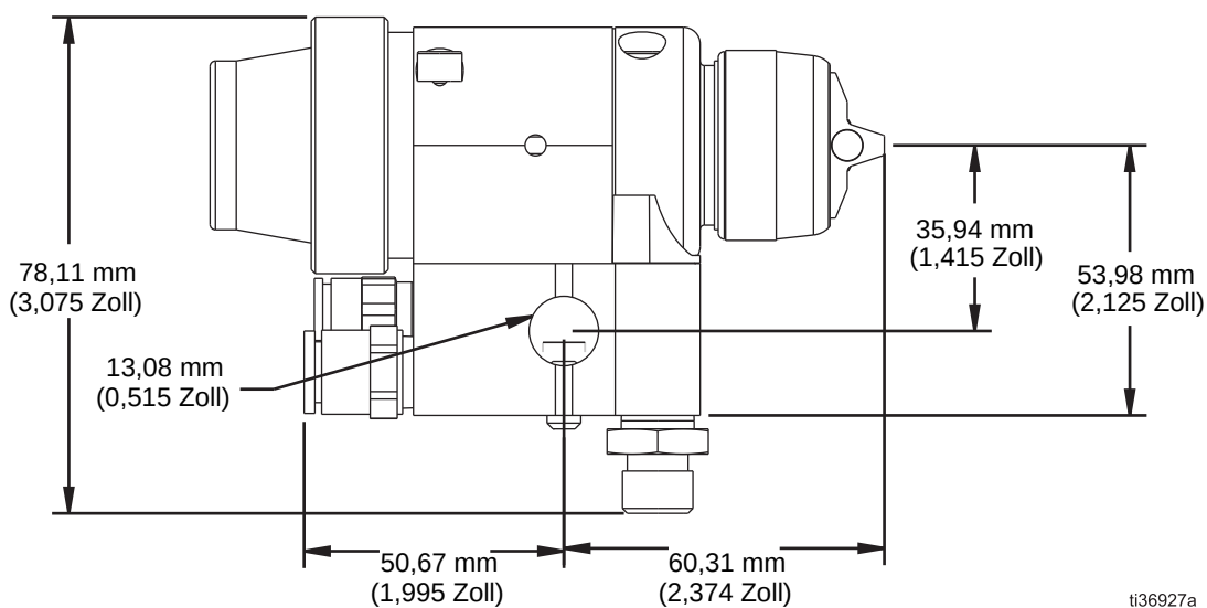
ABB. 30: Montagebohrungen
