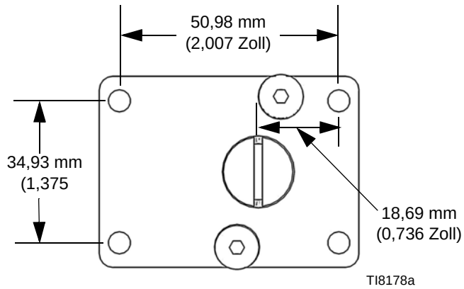
ABB. 26: Montagebohrungen
