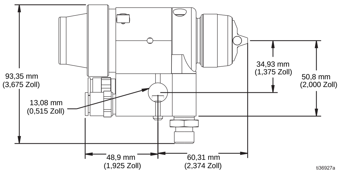
ABB. 29: Montagebohrungen
