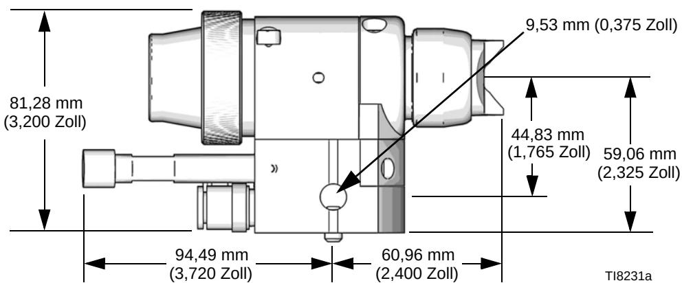
ABB. 27: Montagebohrungen
