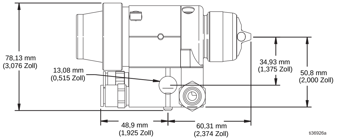
ABB. 28: Montagebohrungen
