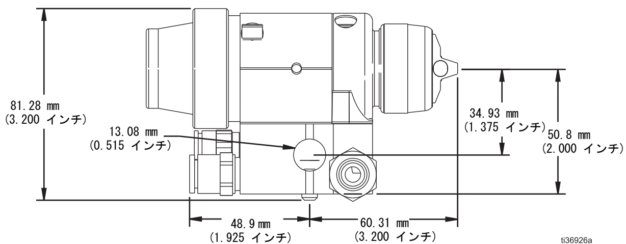
図 28: 取り付け穴の配置
