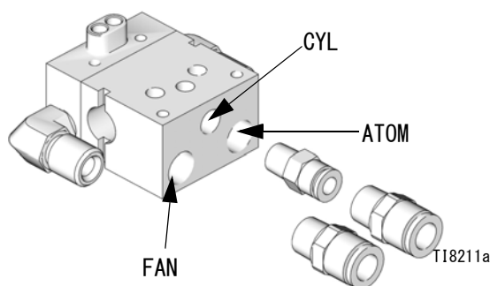
図 2: エア取り付け金具
