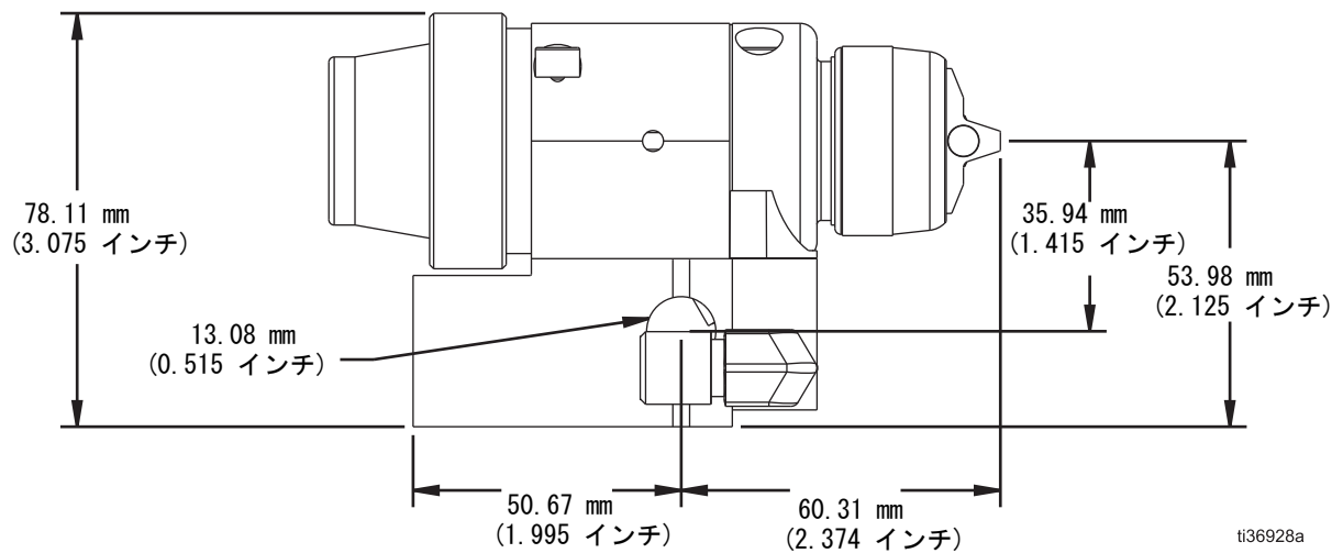
図 30: 取り付け穴の配置
