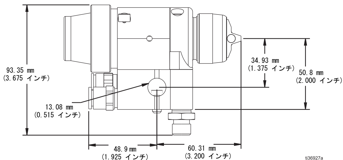
図 29: 取り付け穴の配置
