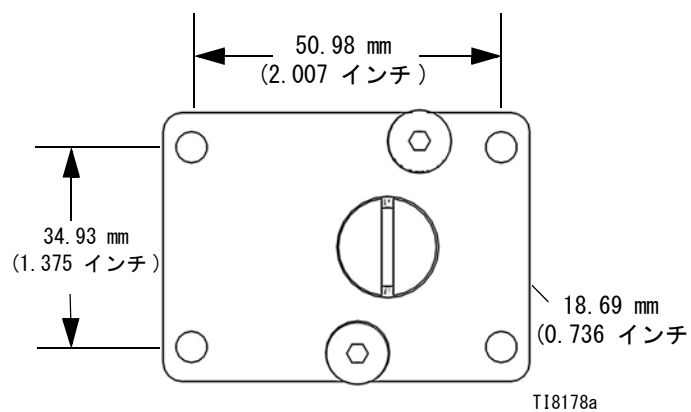
図 26: 取り付け穴の配置
