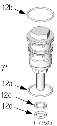
포켓 (12) 상세도
