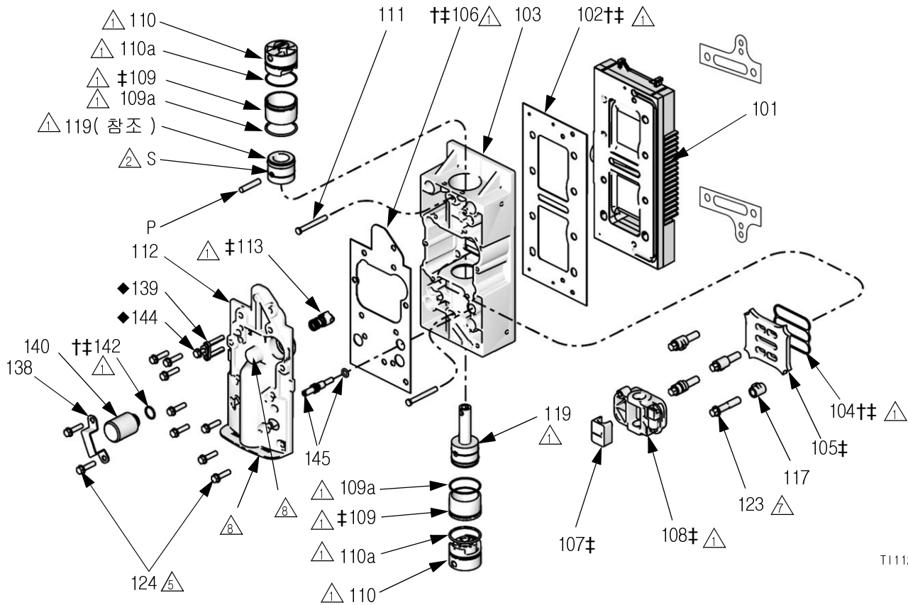
그림 11. 공기 밸브 수리 (그림은 NXT107 임 )
