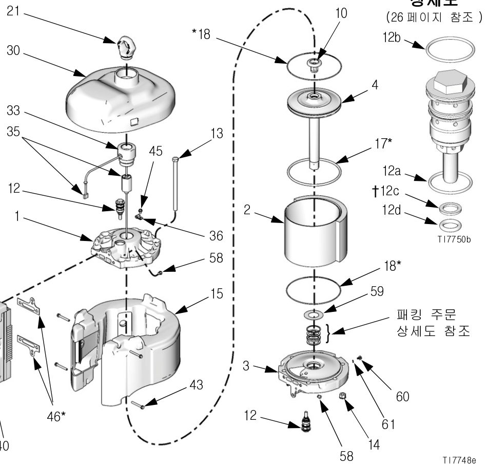
포켓 (12) 상세도
