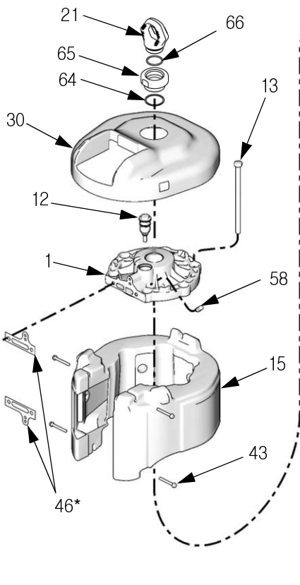
DataTrak 이 없는 모델의 상단 덮개 (30) 상세도
