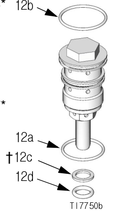
포켓 (12) 상세도 (26 페이지 참조)
