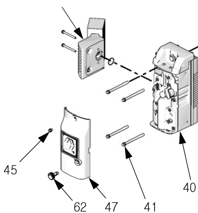
위의 배기장치 상세도 참조
