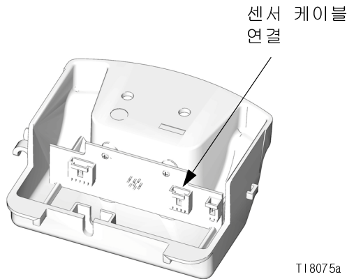
그림 15. 센서 케이블 연결
