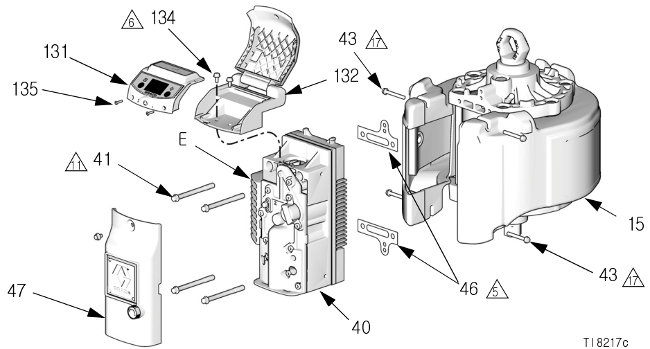
그림 9. 공기 밸브 제거 (DataTrak 모듈이 함께 표시된 모델)
