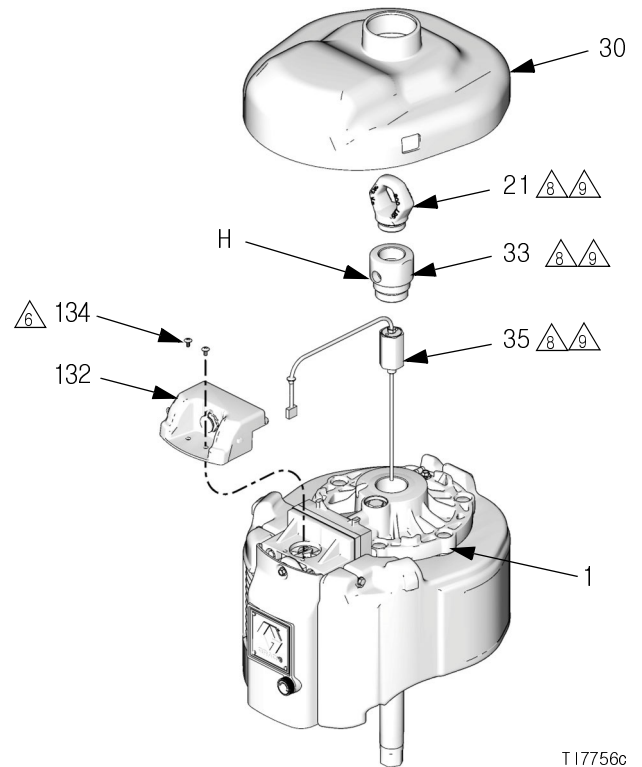
그림 16. 선형 센서 교체
