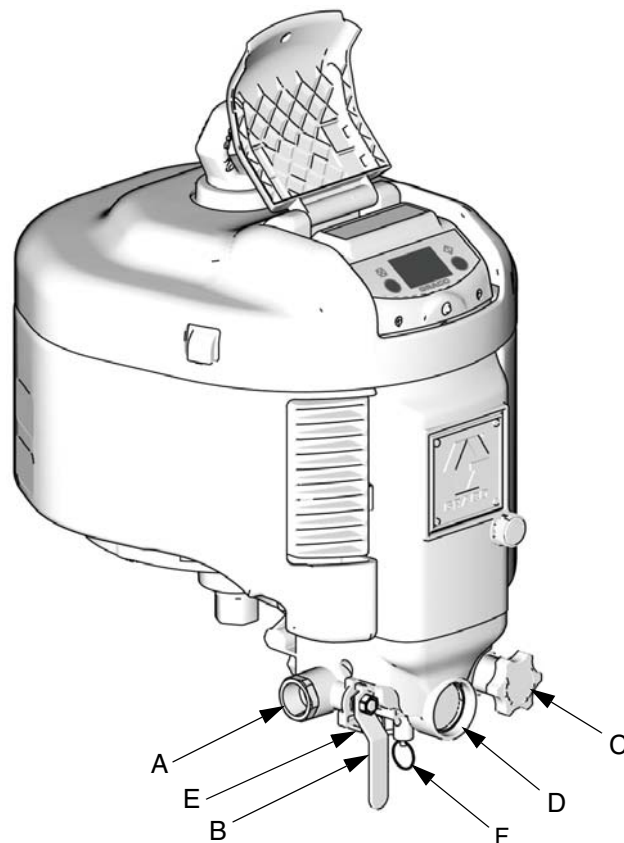
FIG. 1 : Module de commande d'air monté sur le moteur pneumatique NXT
