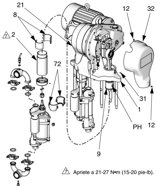
FIG. 6. Kit de cilindro de corredera
