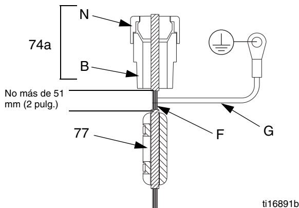
FIG. 30. Circuito del cable de campo de IS
