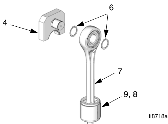
FIG. 19. Brazo de manivela y varilla de conexión
