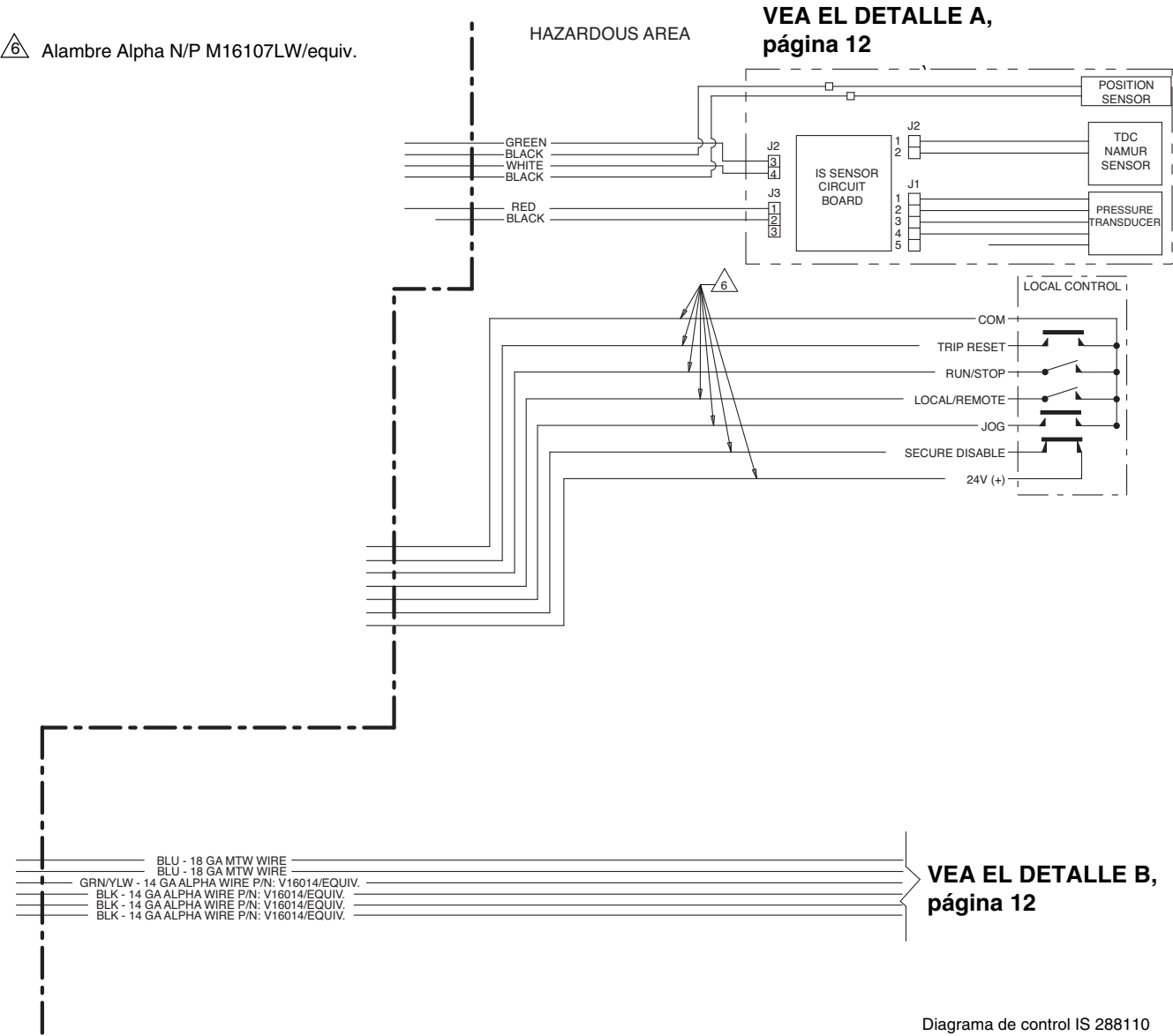
FIG. 2: Diagrama de cableado del sistema, para ubicaciones peligrosas
