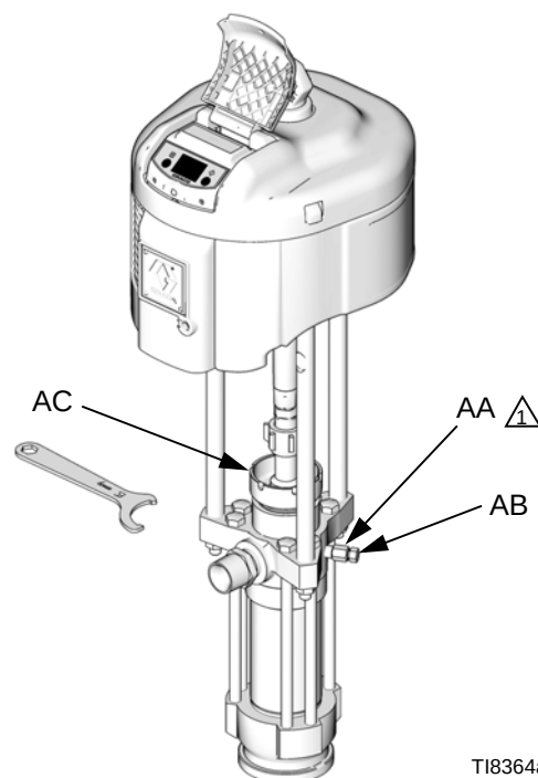
FIG. 3. Valvola di spurgo e tazza del liquido
