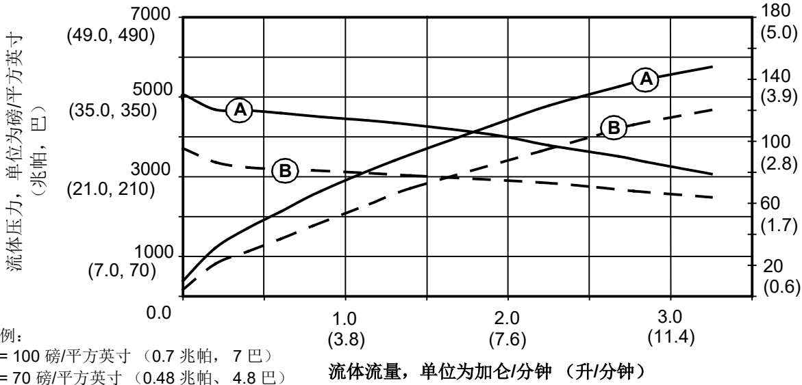
XM50 流体性能和空气消耗量
