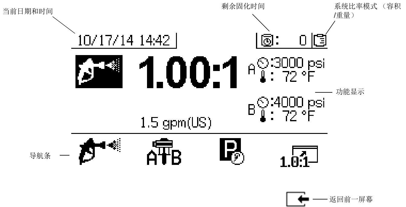
图 6: 主显示屏的部件 (所示为所有显示功能均启用)
