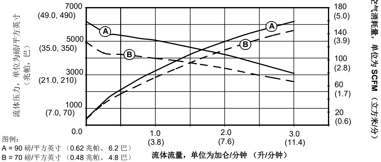
XM70 流体性能和空气消耗量
