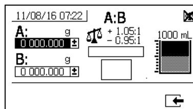
系统比率模式（按重量）
