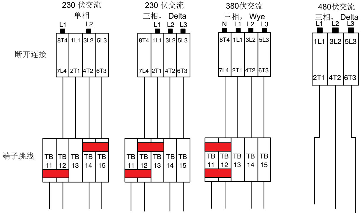
图 7: XM 接线图
