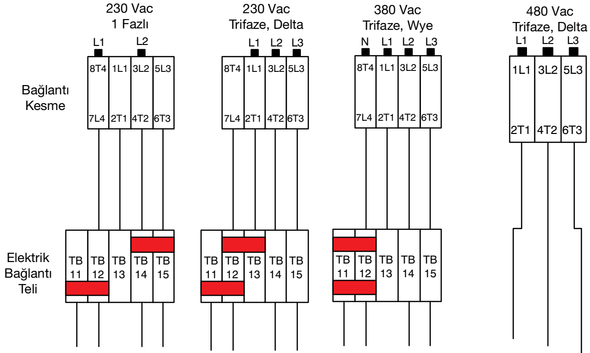
ŞEKİL 7: XM Kablo Tesisat Şeması
