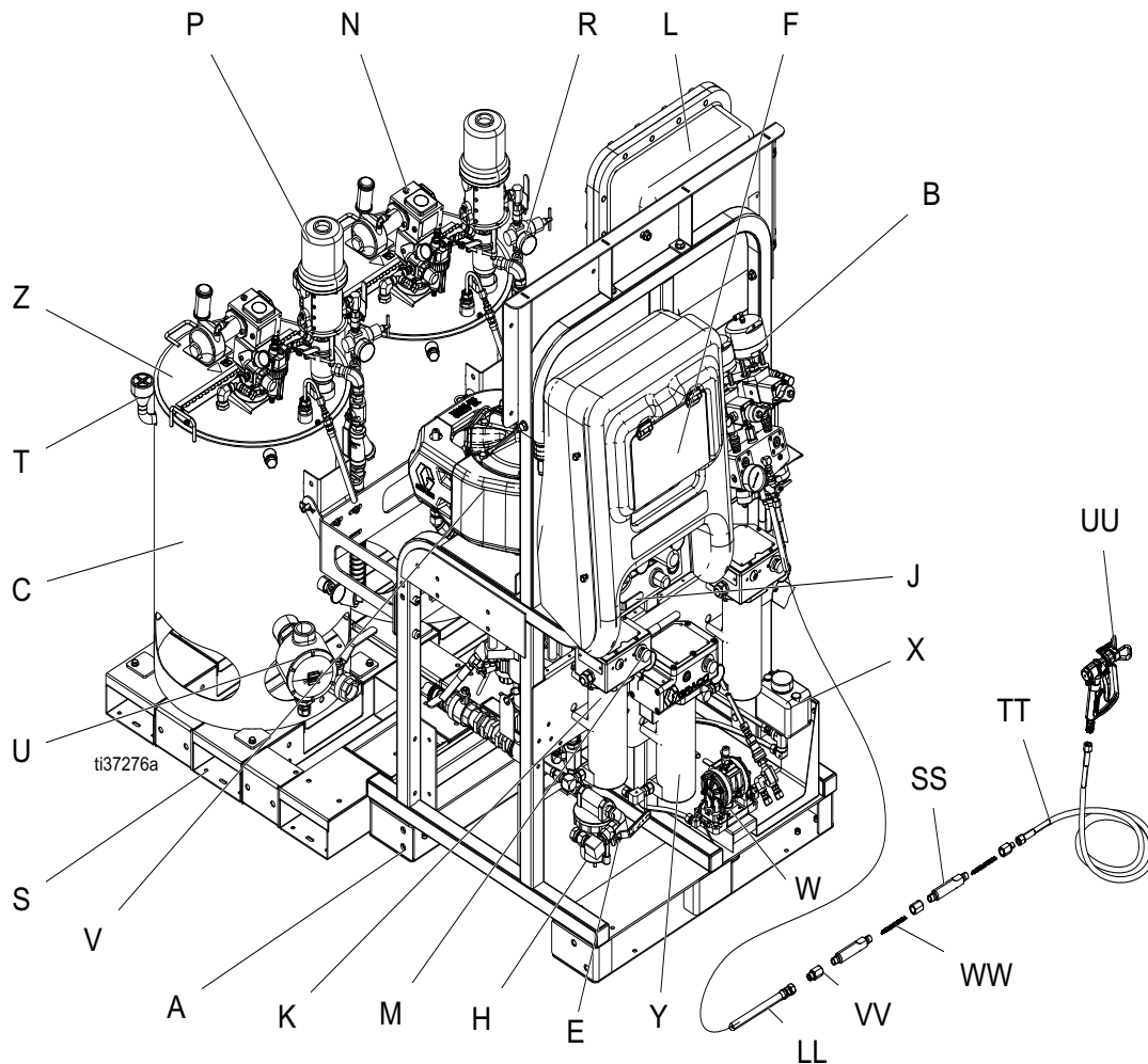
FIG. 1: Configurație tipică: Rezervor de 25 de galoane cu pereți dubli, cu recirculare (vedere frontală)
