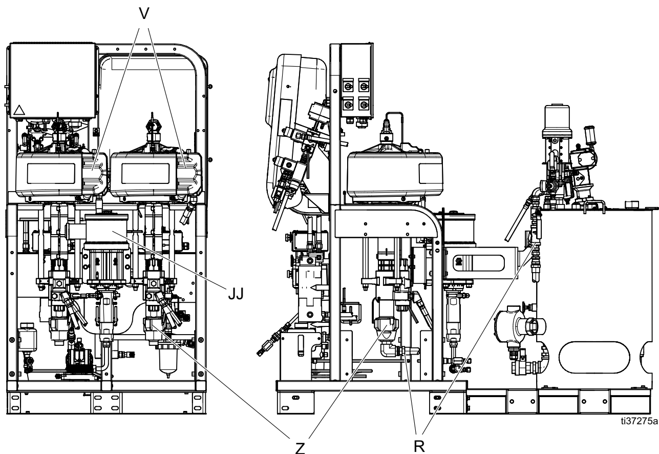
FIG. 2: Configurație tipică: Rezervor de 25 de galoane cu pereți dubli, cu recirculare (vedere din spate și laterală)
