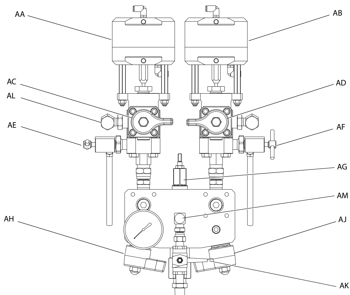
FIG. 3: Ansamblu de control al fluidului
