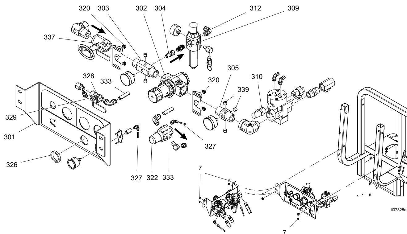
FIG. 1 Commandes pneumatiques
